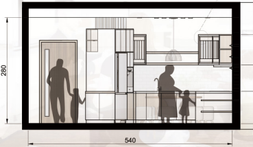
A-A剖面圖 S=1:30 單位:cm
