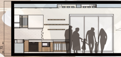
D-D剖面圖 S=1:30 單位:cm
