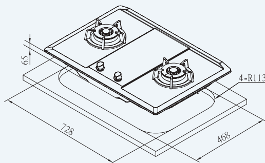
G2623S
