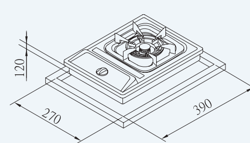
G251KE
