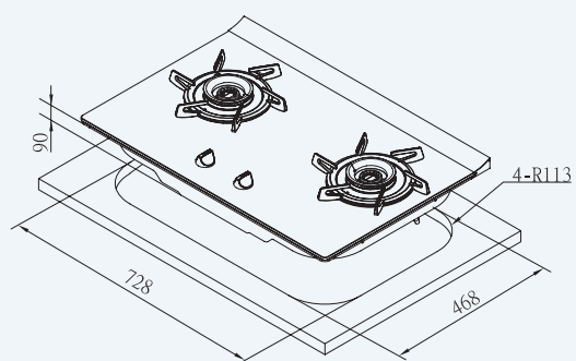
G2921G
