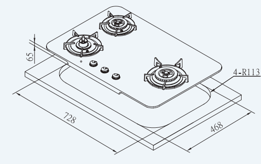
G2830KGB
