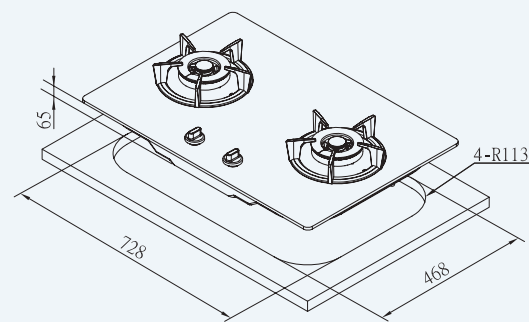
G2623AG
