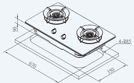
G2923AG
