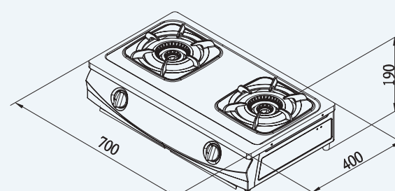
G5513S
