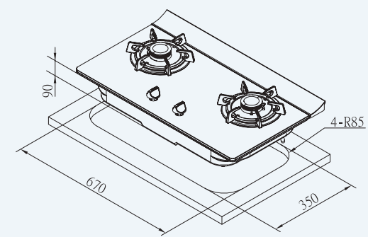
G2826G
