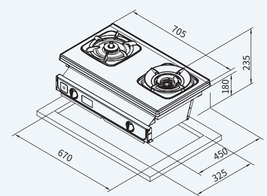
G6920AS
