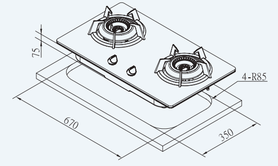
G2721G
