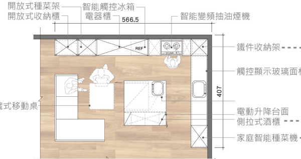
平面配置圖 S=1/30
